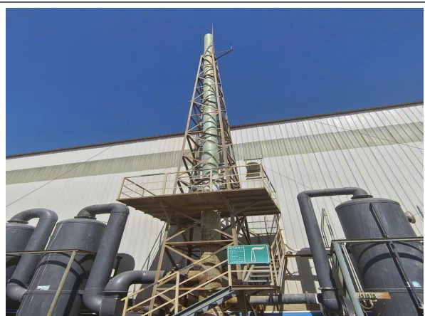
废气排放口
